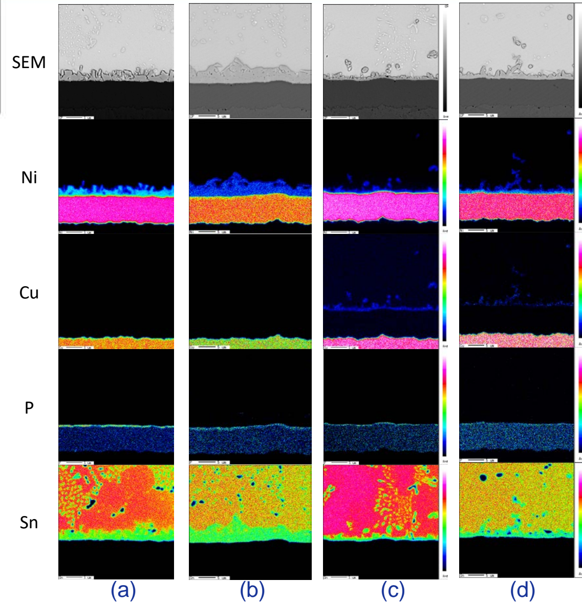
a) SABI-T0 b) SABI- 500TC c) SABIX-T0 d) SABIX-500TC
